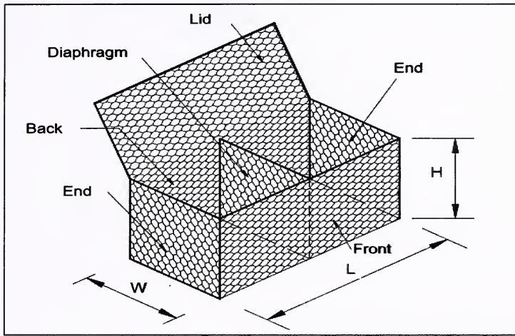
Fig. A- Gabion Box
